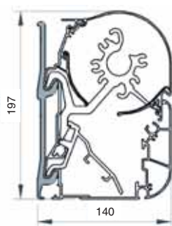
Uchycení boční
