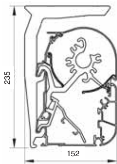
Uchycení stropní
